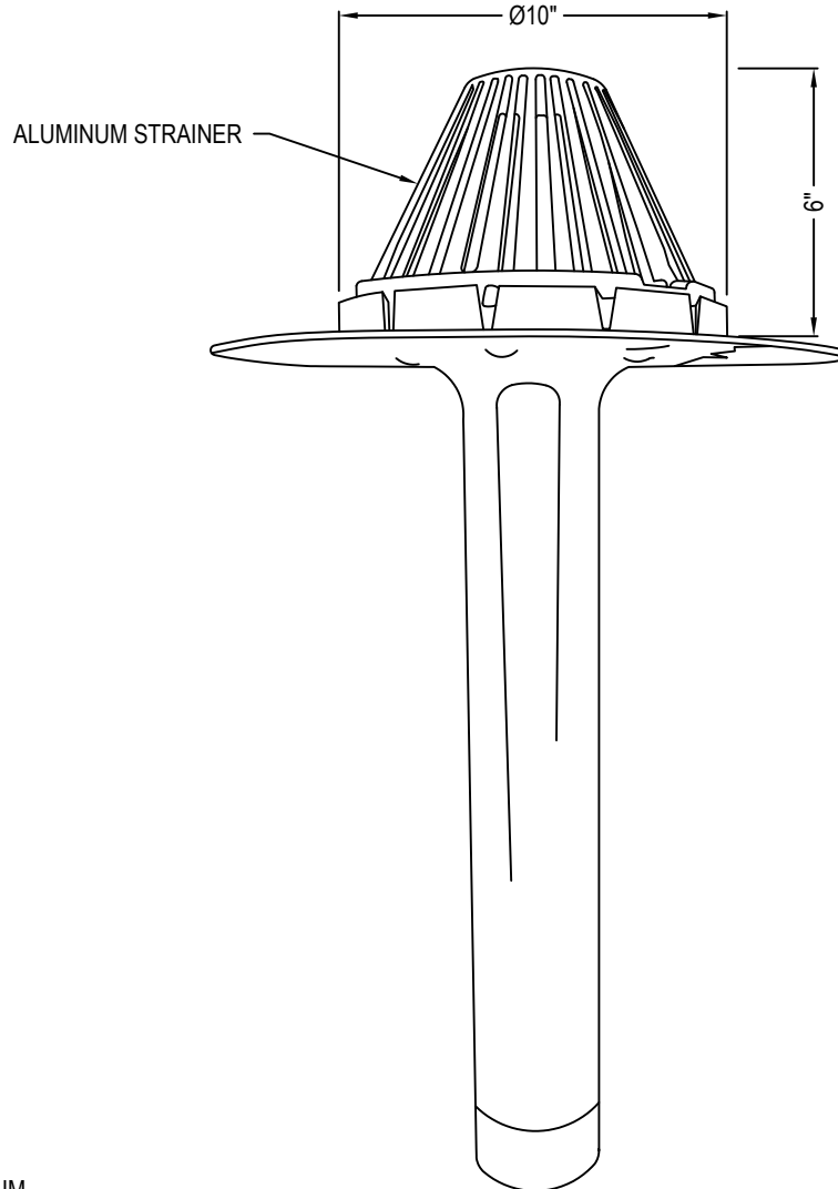
ELEVATION
